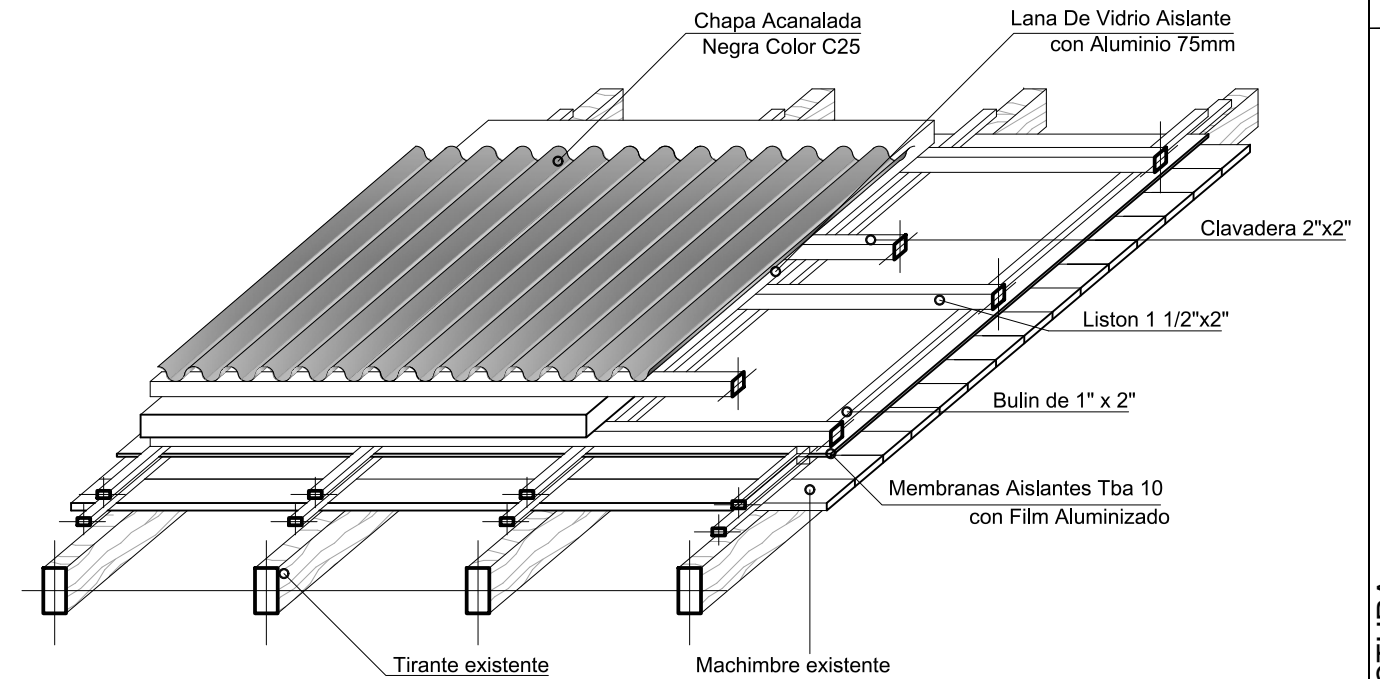
Detalle de Cubierta ① Esc. 1.25
