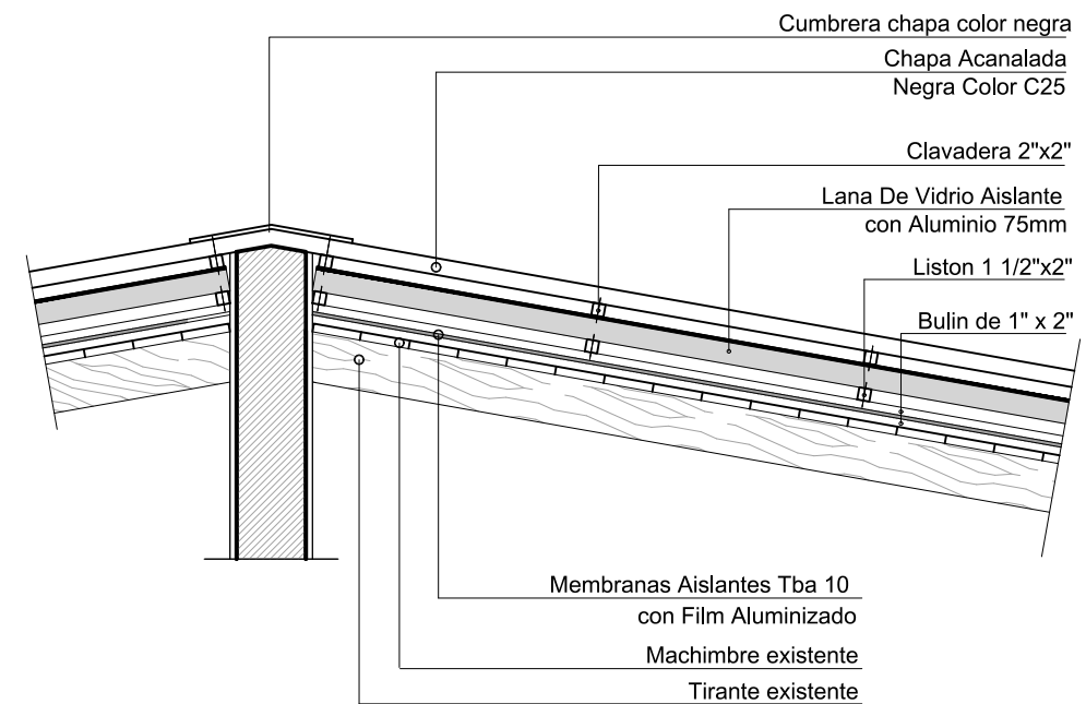
Detalle de Cubierta ② Esc. 1.25
