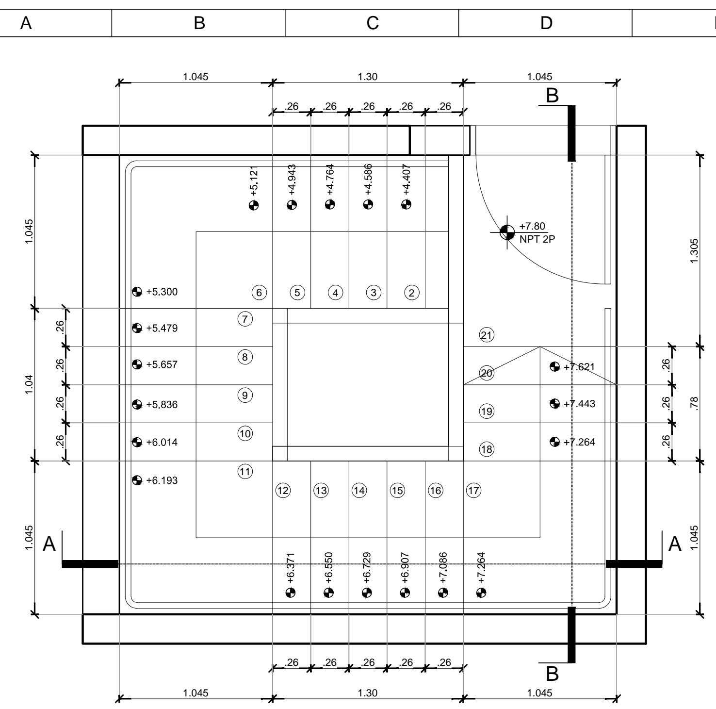
PLANTA 2º PISO
