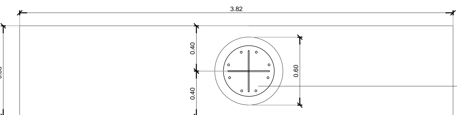
PLANTA DE APOYO INFERIOR ESC.1.20
