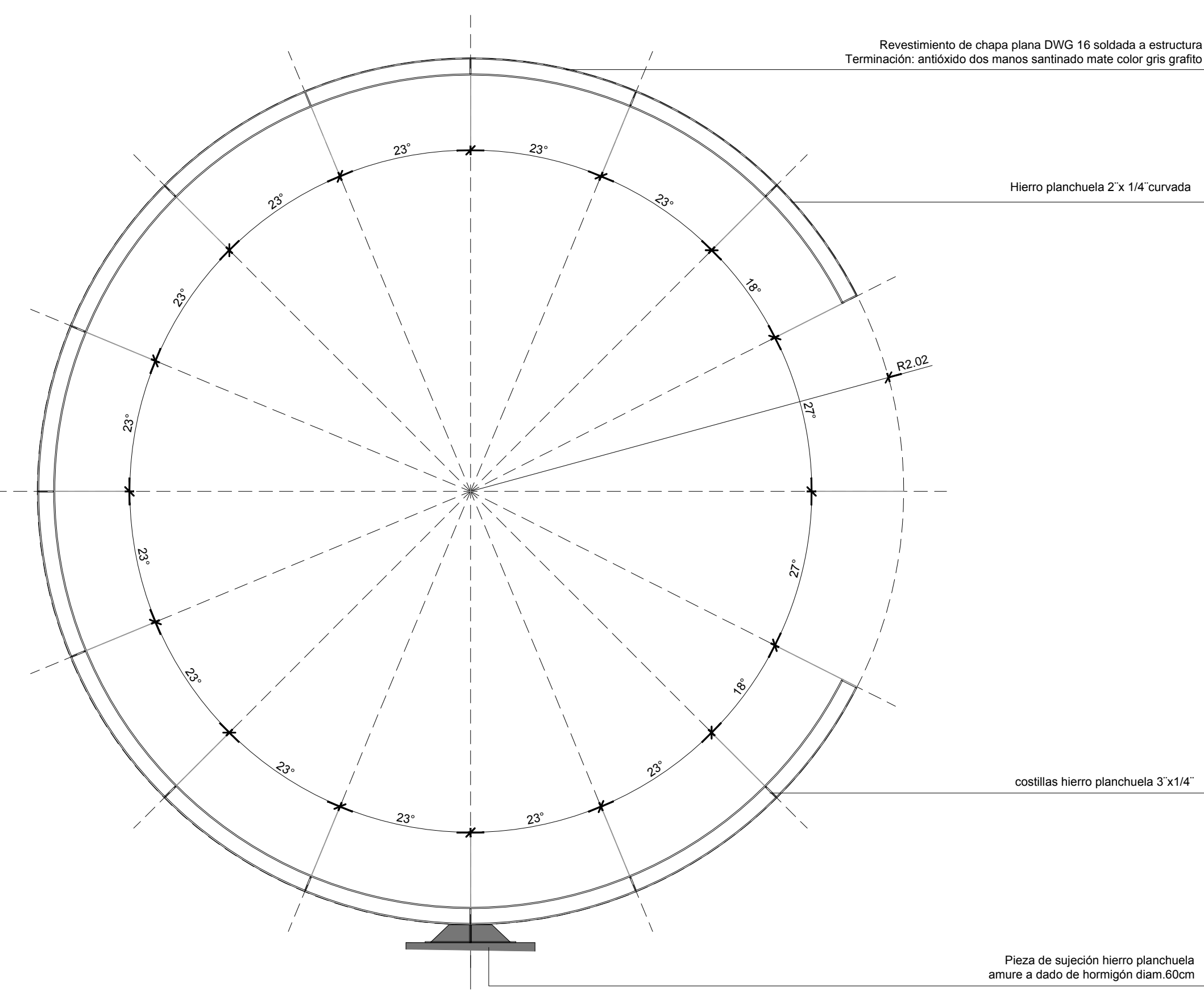
VISTA ESTRUCTURA ESC.1.20
