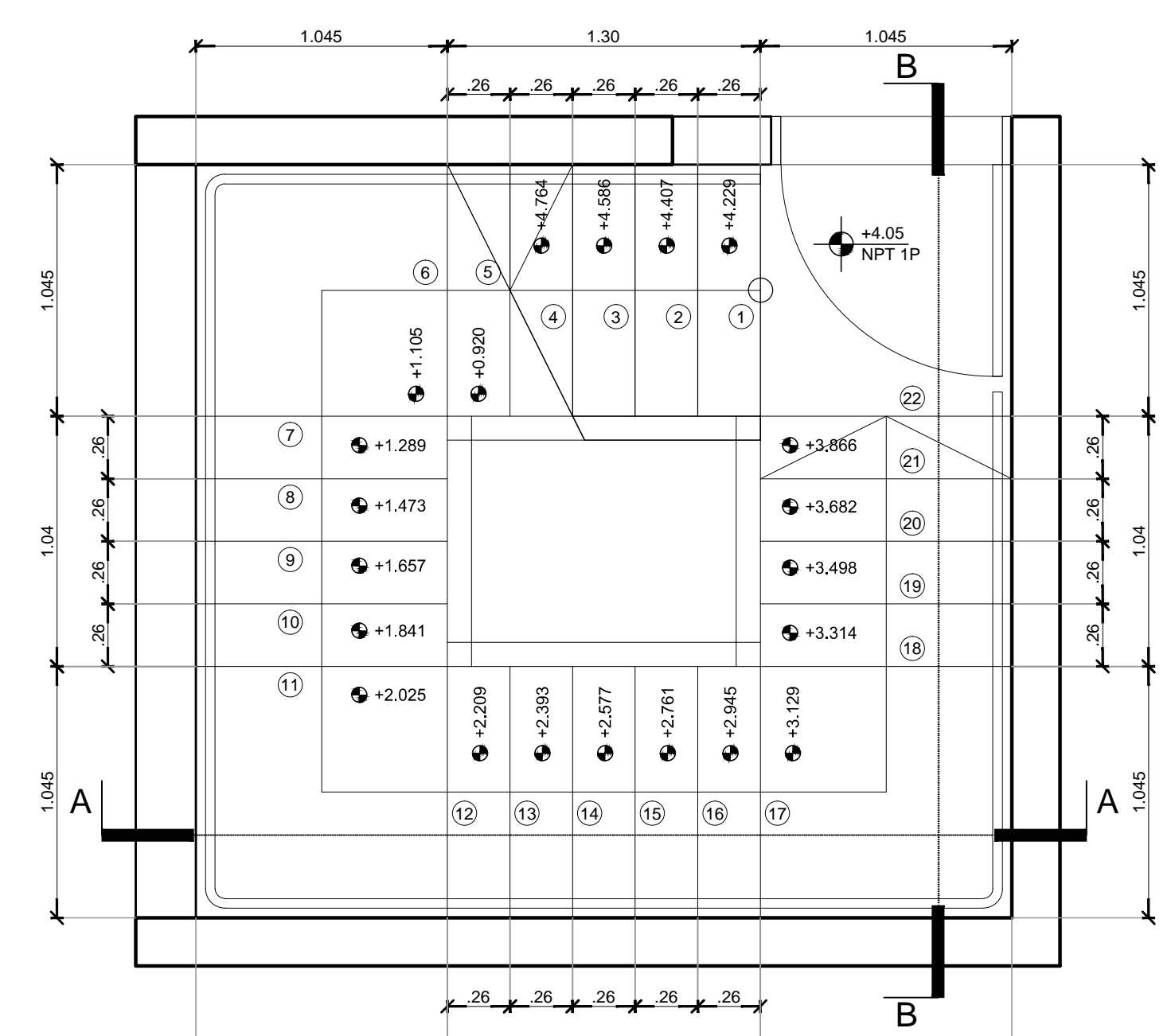
PLANTA 2º PISO
