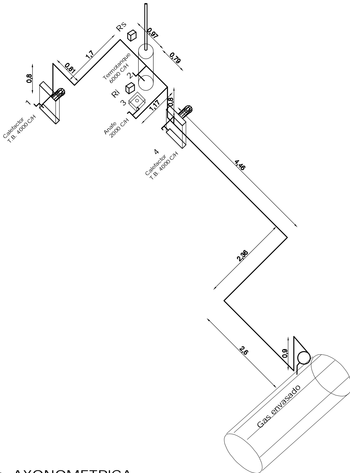
Vista: AXONOMETRICA
