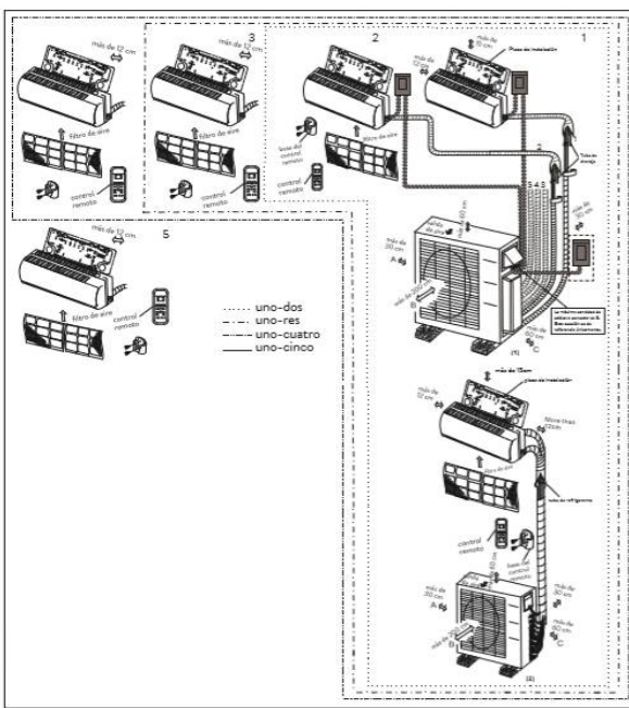
DIAGRAMA DE INSTALACIÓN
