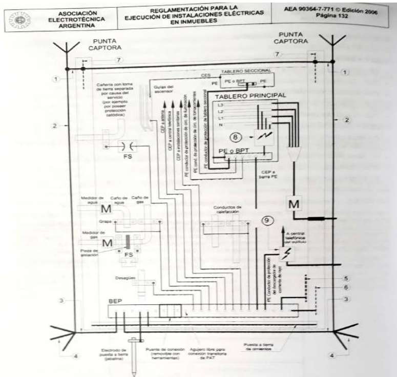
Figura 771.16.D – Equipotencialización típica en un esquema de conexión a tierra TT donde: 1: interconexión equipotencial entre los conductores de bajada del sistema de protección contra descargas atmosféricas de acuerdo con IEC 62305. 2: conductores de bajada del sistema de protección contra descargas atmosféricas. 3: interconexión equipotencial entre las puestas a tierra de descargas atmosféricas y la tierra de protección. 4: electrodos de puesta a tierra del sistema de protección contra descargas atmosféricas (simbolizados en la clásica ejecución de pata de ganso). 5: estructura metálica del edificio (si existe) equipotencializada a tierra. 6: armadura del hormigón armado equipotencializada a tierra. 7: interconexión equipotencial entre los conductores de bajada del sistema de protección contra descargas atmosféricas y las armaduras del hormigón armado de acuerdo con IEC 62305. 8: dispositivo de protección contra las sobretensiones (eventualmente descargador de corriente de rayo) para la alimentación. 9: dispositivo de protección contra las sobretensiones para las líneas telefónicas.
