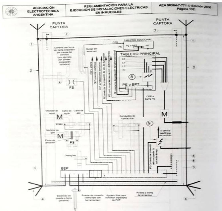
Figura 771.18.D – Equipotencialización típica en un esquema de conexión a tierra TT donde: 1: interconexión equipotencial entre los conductores de bajada del sistema de protección contra descargas atmosféricas de acuerdo con IEC 62305. 2: conductores de bajada del sistema de protección contra descargas atmosféricas. 3: interconexión equipotencial entre las puestas a tierra de descargas atmosféricas y la tierra de protección. 4: electrodos de puesta a tierra del sistema de protección contra descargas atmosféricas (simbolizados en la clásica ejecución de pata de ganso). 5: estructura metálica del edificio (si existe) equipotencializada a tierra. 6: armadura del hormigón armado equipotencializada a tierra. 7: interconexión equipotencial entre los conductores de bajada del sistema de protección contra descargas atmosféricas y las armaduras del hormigón armado de acuerdo con IEC 62305. 8: dispositivo de protección contra las sobretensiones (eventualmente descargador de corriente de rayo) para la alimentación. 9: dispositivo de protección contra las sobretensiones para las líneas telefónicas.
