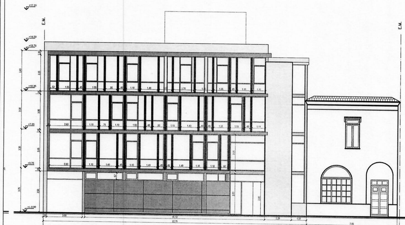
VISTA FRENTE sobre calle MORENO
